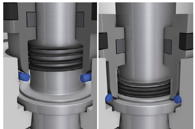
Automatische Spindelarreterung – patentiertes System für eine immer exakte Bohrtiefe bei unterschiedlichen Werkstoffen. Mit Drehzahlen von 1500–7500 1/min für hohe Vorschübe bzw. kurze Bohrtakte.
